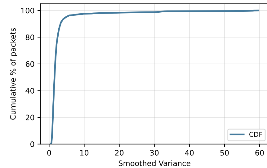
(d) CDF — Smoothed Variance
